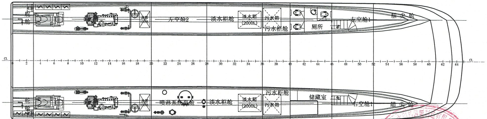
舱底布置图
